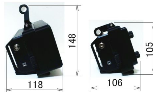
「アイコミック705/905」装着・側面寸法
