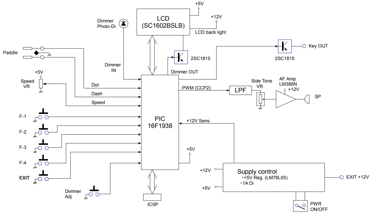
図1 回路ブロック
